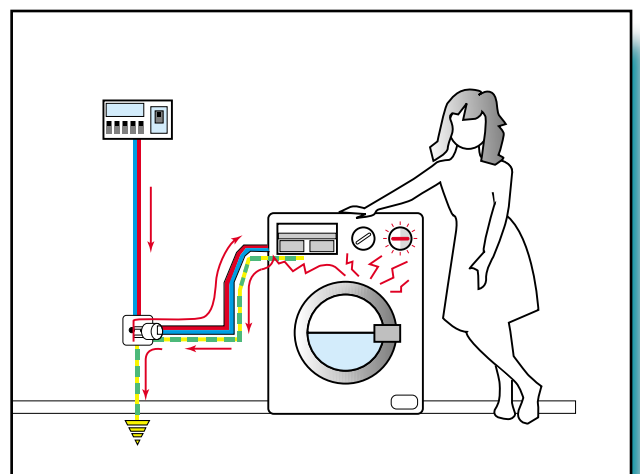
Avec prise de terre et disjoncteur différentiel
