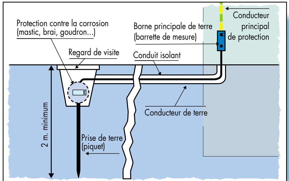
Conducteurs verticaux
